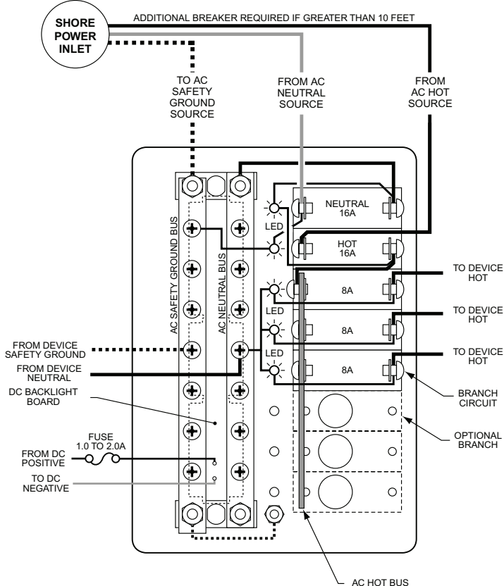
Wiring Diagram AC Master Panel PN 8127 / PN 3127
